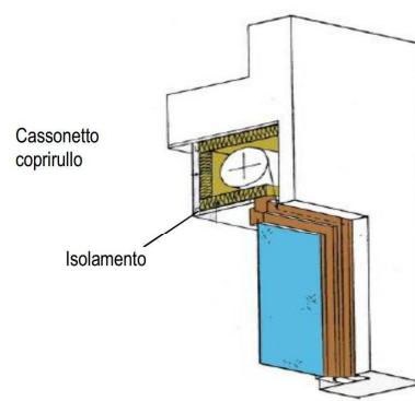
Isolamento del cassonetto dell'avvolgibile
